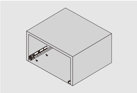
Закрепите направляющие на корпус
