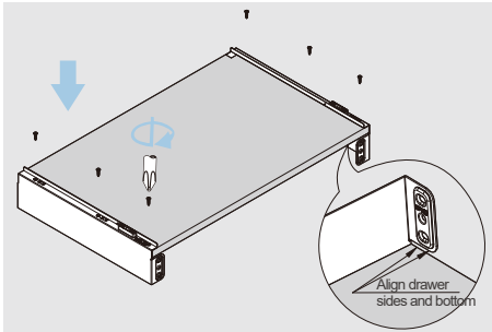
Выровняйте боковины и дно ящика, зафиксируйте винты и соберите дно.
