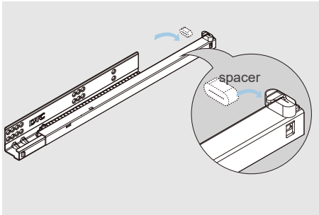
Установите проставку на задний крючок направляющей
