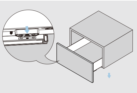
Установите ящик на направляющую
